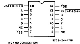
CD4002B
