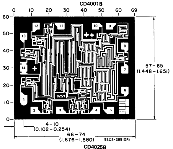
CD4025B
