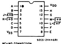
CD4001B
