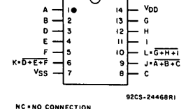
CD4025B
