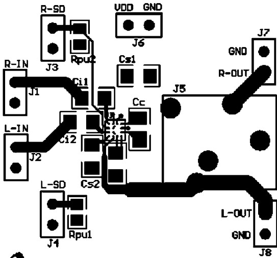
Top Layer
