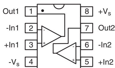
SOIC
