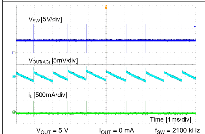
Figure 24. PFM Mode
