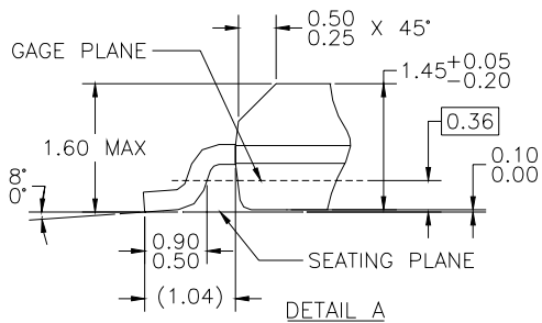
SCALE: 24:1
