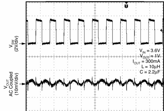
Ripple
