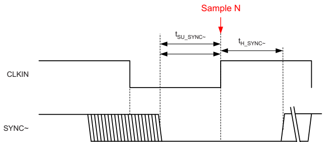
Figure 147. SYNC~ Timing (Subclass 2)
