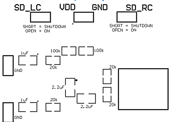
Top Overlay
