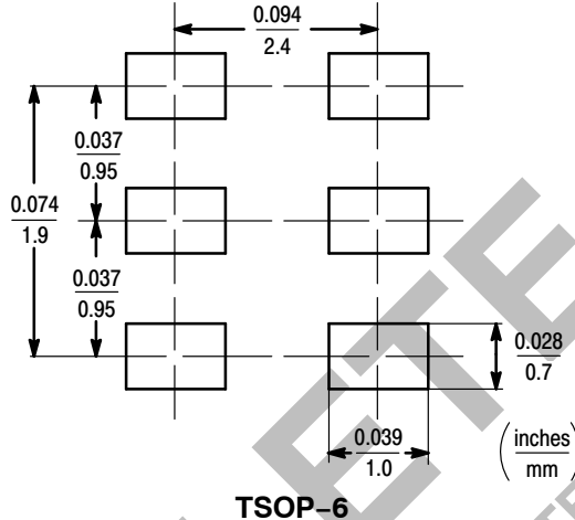
TSOP-6
