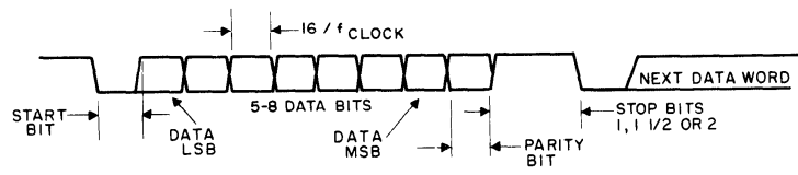
Fig. 12 - Serial data word format.
