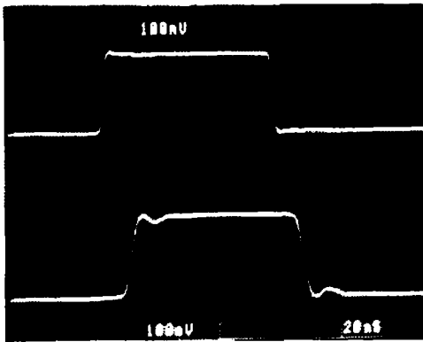
Vertical Scale: V_{IN} = 100\text{mV/Div.} , V_{OUT} = 100\text{mV/Div.} Horizontal Scale: 20\text{ns/Div.}
