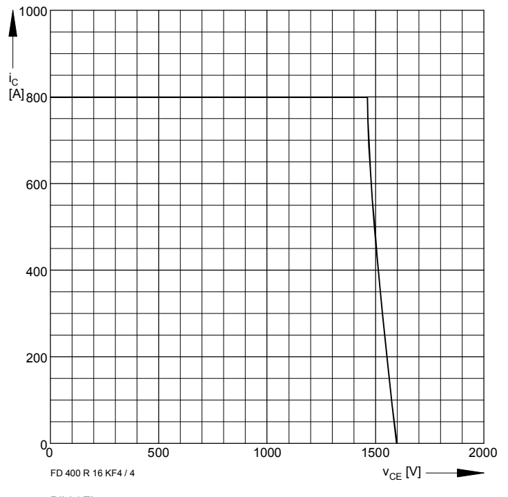
Bild / Fig. 4 Rückwärts-Arbeitsbereich / Reverse biased safe operating area t_{vj} = 125^\circ\text{C} v_{LF} = v_{LR} = 15 \text{ V} R_G = 4,7 \Omega
