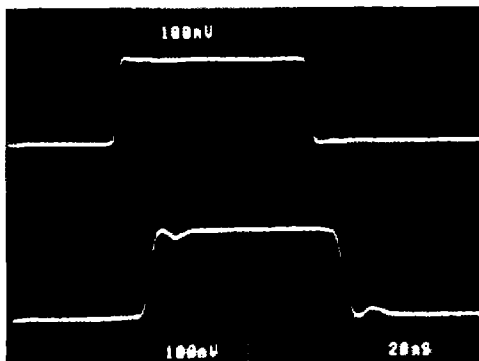
Vertical Scale: V_{IN} = 100mV/Div. , V_{OUT} = 100mV/Div. Horizontal Scale: 20ns/Div.
