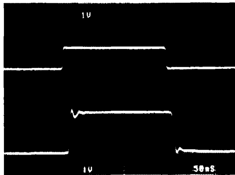
Vertical Scale: V_{IN} = 1V/Div. , V_{OUT} = 1V/Div. Horizontal Scale: 50ns/Div.
